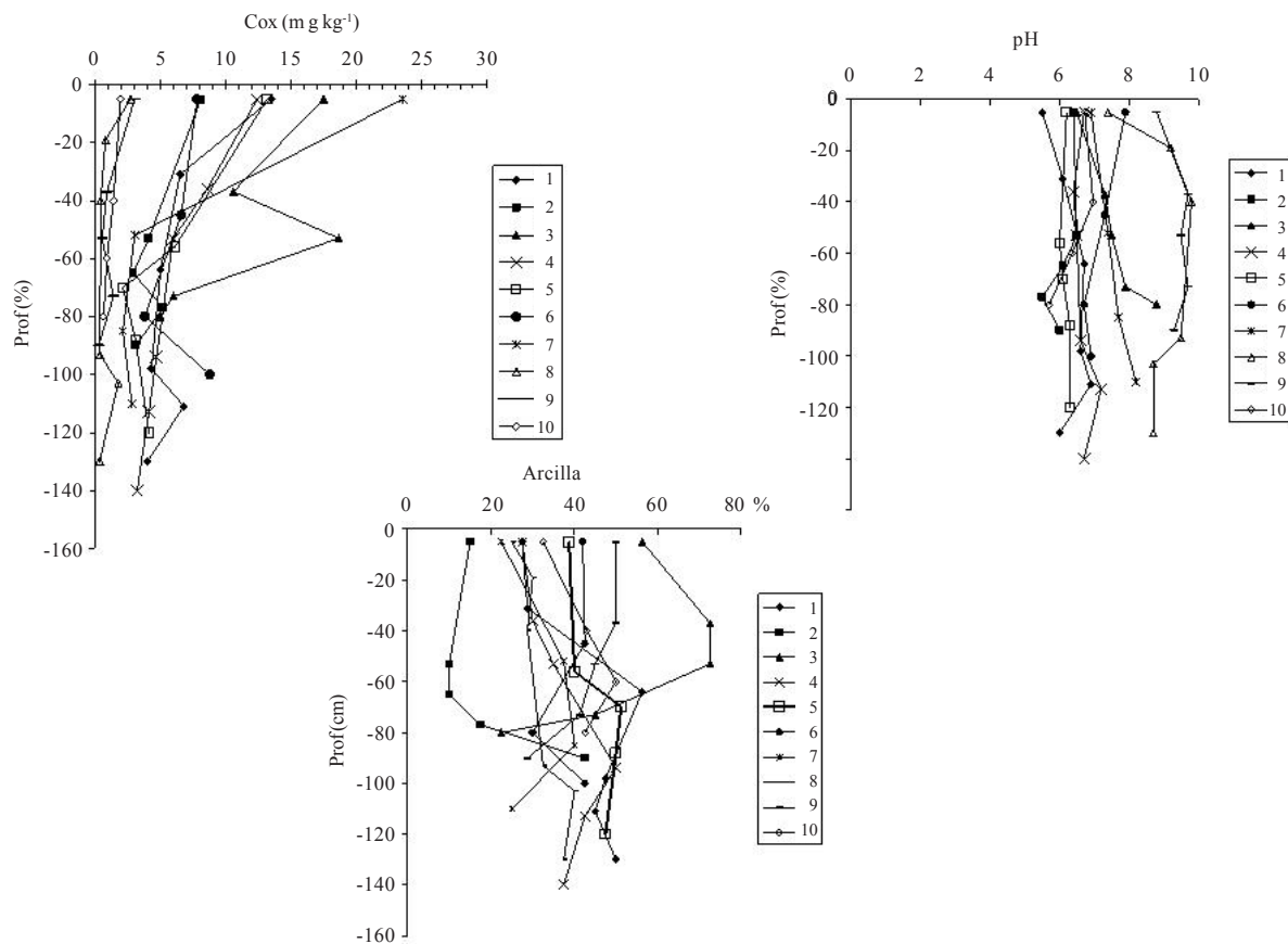
Figura 2. Perfiles de Cox, pH y arcillas para todos los suelos evaluados.
